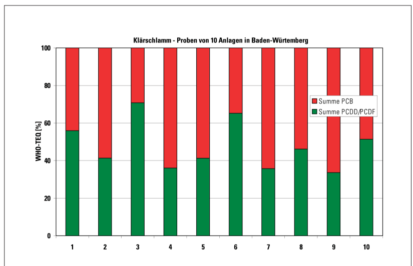
Abb. 16: TEQ Verteilung auf PCB und PCDD/PCDF von Klärschlämmen aus kommunalen Kläranlagen – Baden-Württemberg
