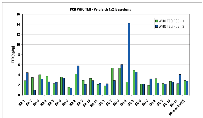
Abb. 15: Vergleich der PCB WHO TEQ der beiden Probenahmen an 22 bayerischen Kompostierungsanlagen 2002
